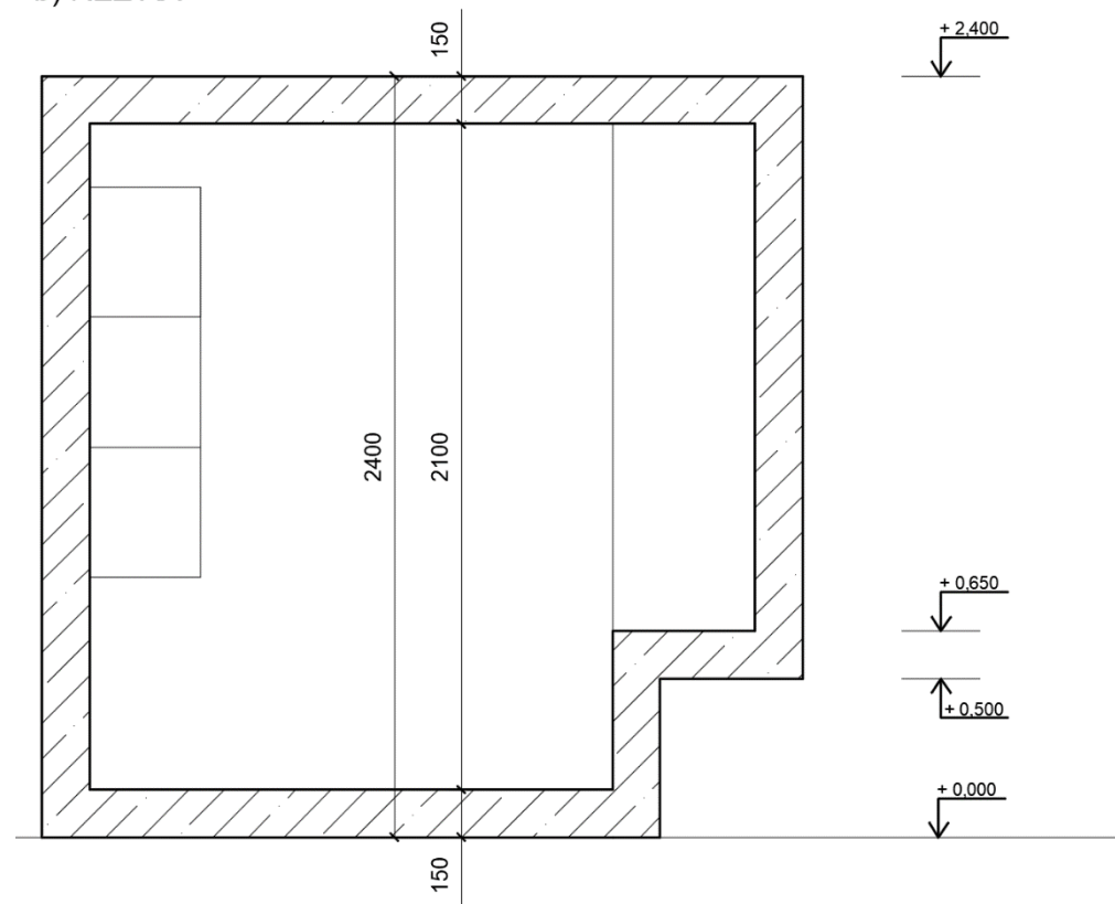
b) ŘEZ AA'
