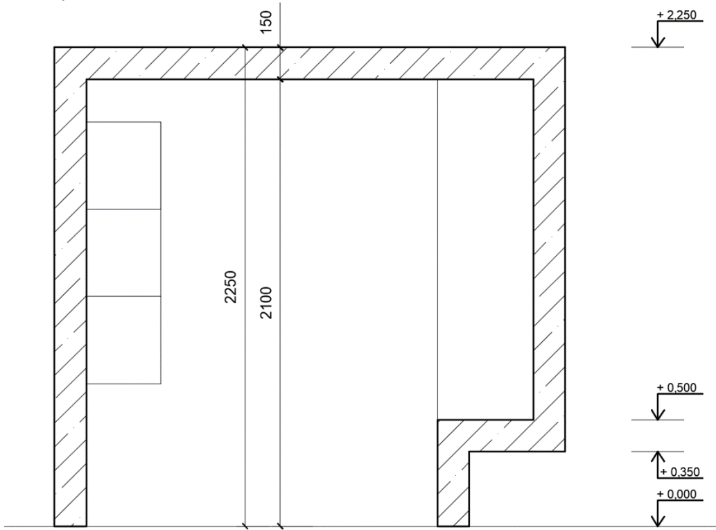
a) ŘEZ AA'
