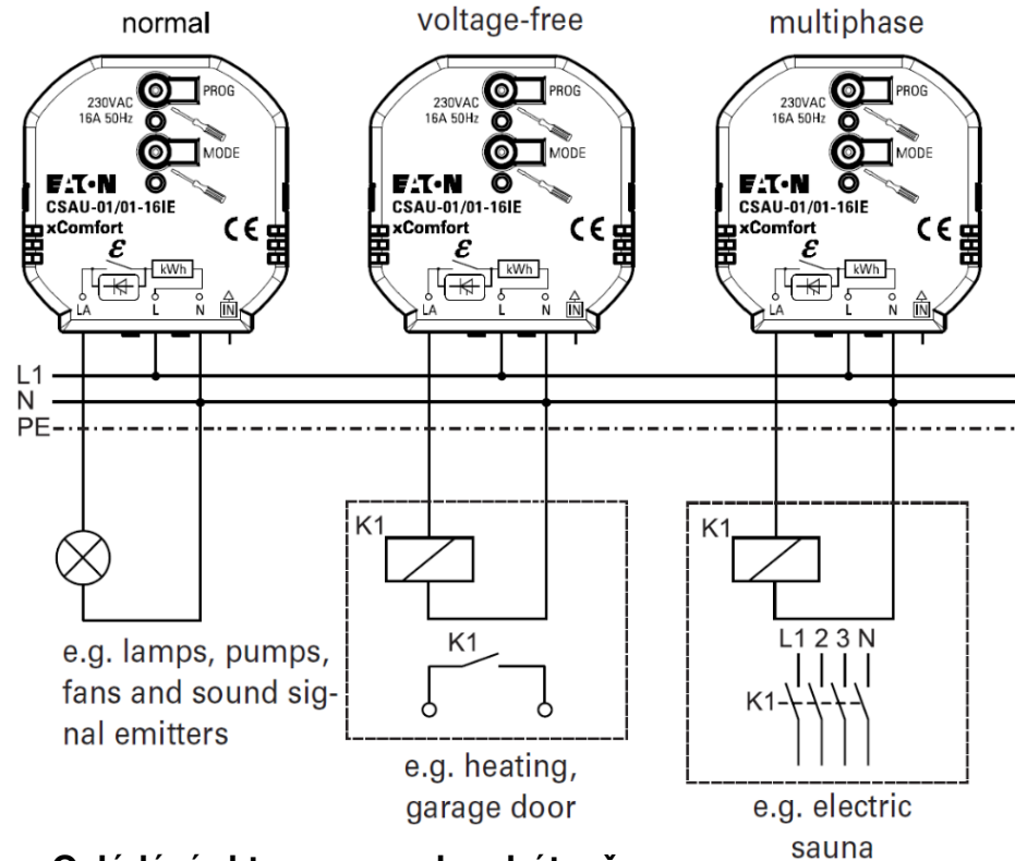
Ovládání aktoru pouze bezdrátově
