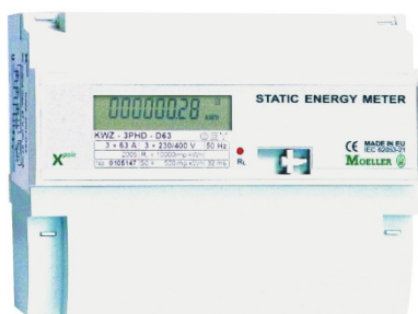
Elektroměr
